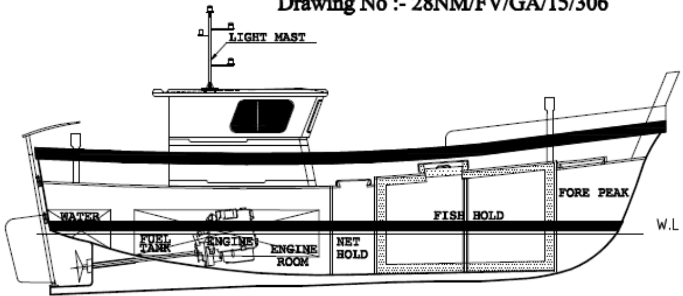
ELEVATION
